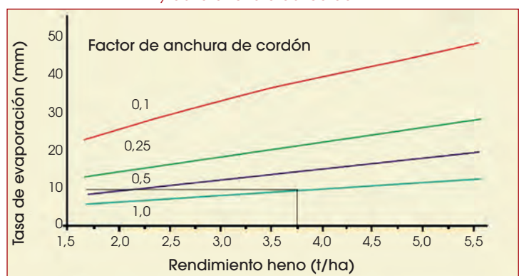
Figura 9. Evaporación total necesaria para secar alfalfa desde el 80% hasta el 20% de humedad en función del rendimiento del cultivo y de la anchura del cordón.
